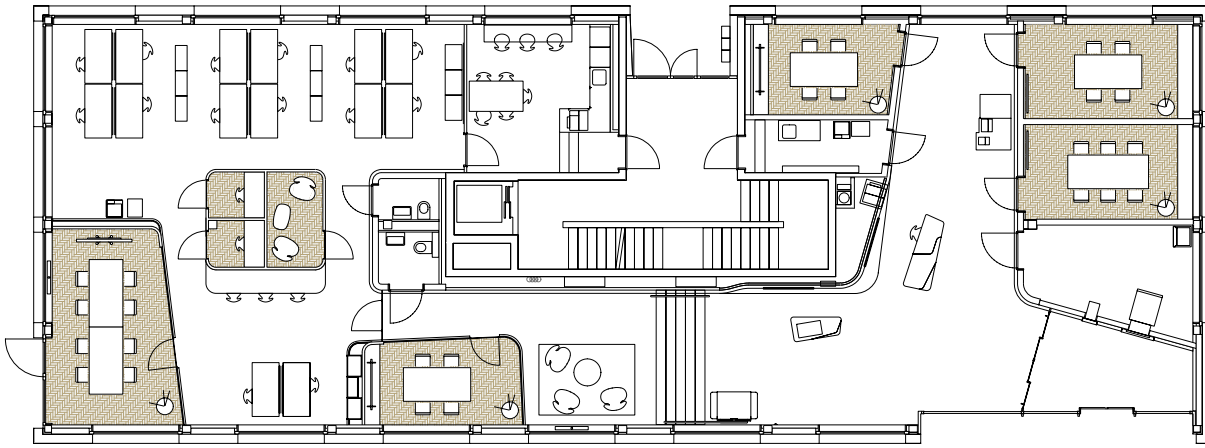
Grundriss Erdgeschoss
