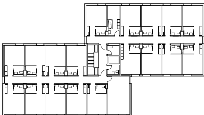
Grundriss Obergeschoss
