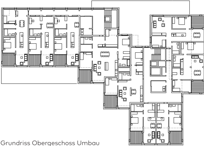
Grundriss Obergeschoss Umbau
