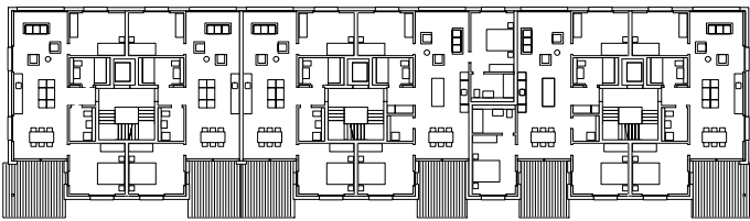
Grundriss Obergeschoss Neubau
